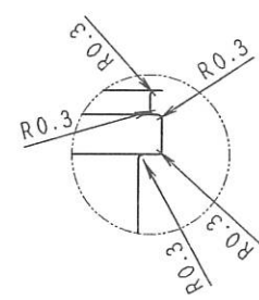
A部詳細 Scale3/1
