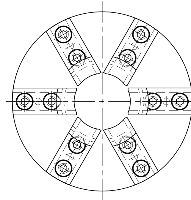
6ヶ取りの場合のレイアウト
